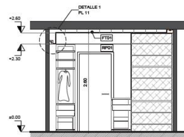
SECCIÓN 3-3
