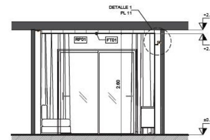
SECCIÓN 4-4
